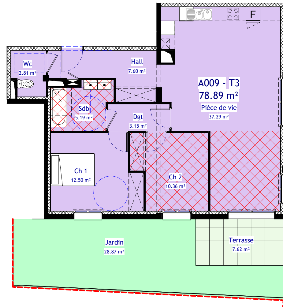
1 PDV A009 - GENERAL Ech : 1 : 100
